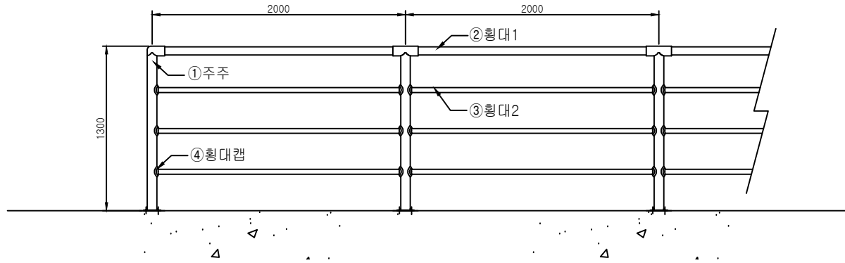
ELEVATION SCALE: NONE
