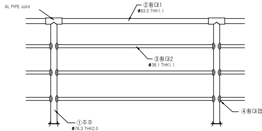
DETAIL SCALE: NONE
