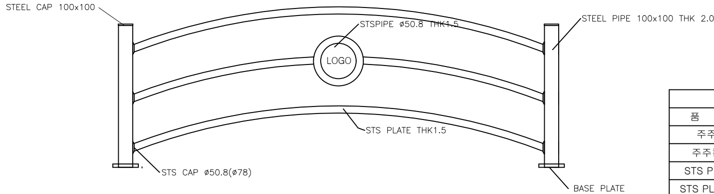
DETAIL SCALE:NONE
