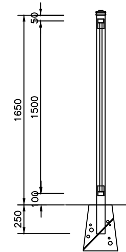
SIDE VIEW SCALE:NONE
