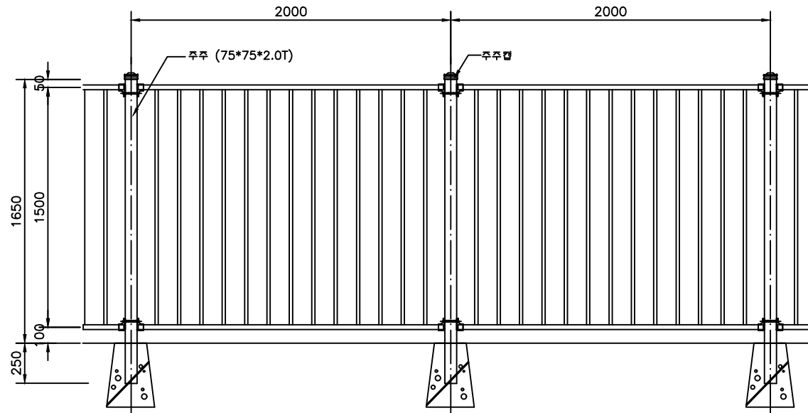
ELEVATION SCALE:NONE
