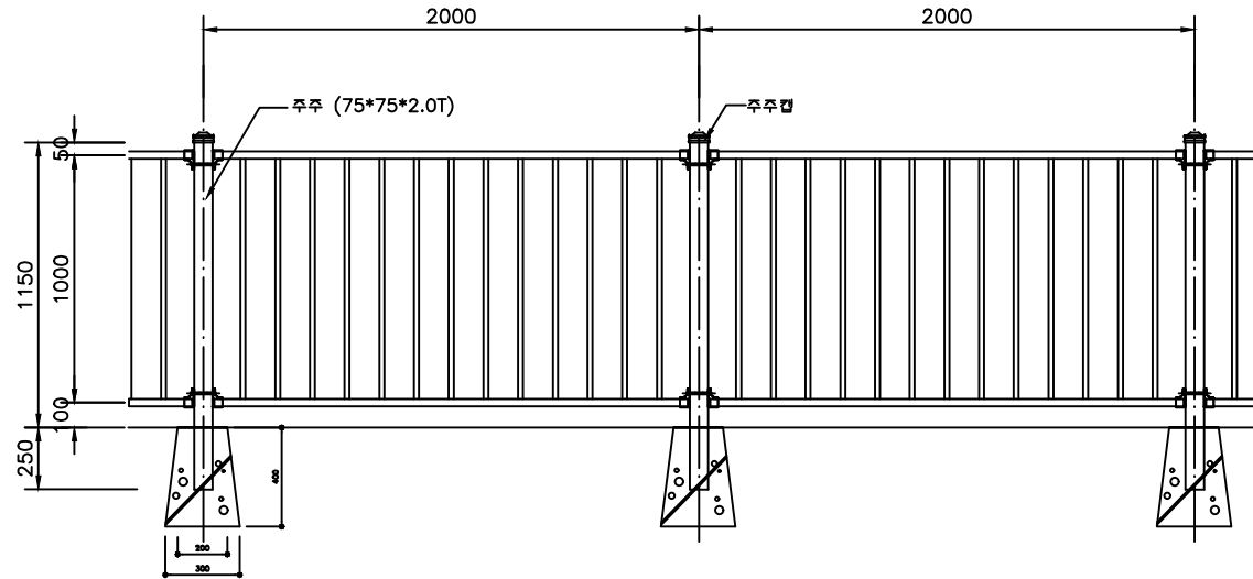
ELEVATION SCALE:NONE
