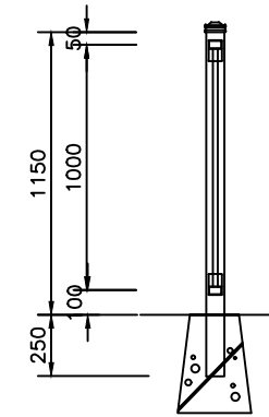
SIDE VIEW SCALE:NONE
