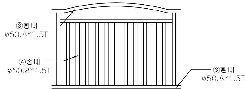
"A" DETAIL SCALE: NONE
