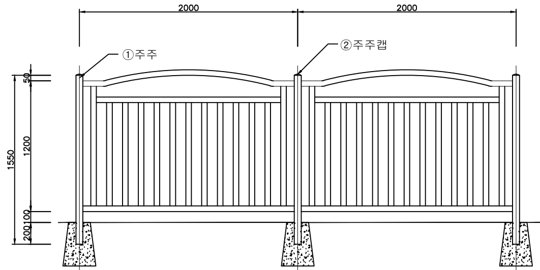
ELEVATION SCALE: NONE
