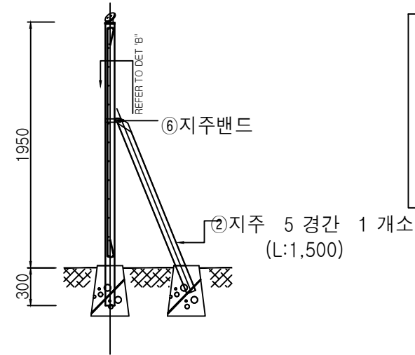
SIDE VIEW SCALE: NONE
