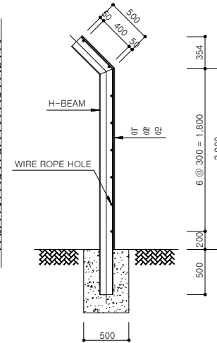
단면도
