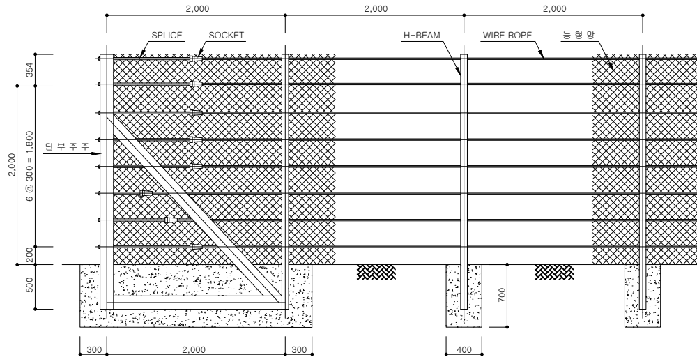
입면도
