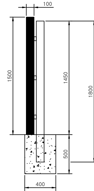
SIDE VIEW SCALE:NONE
