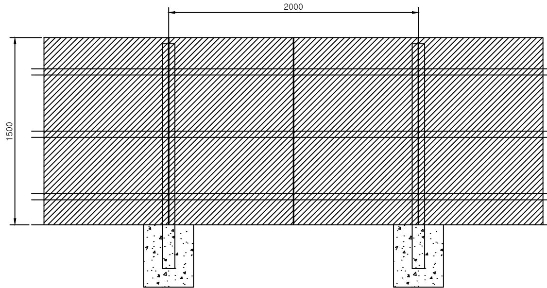
ELEVATION SCALE:NONE
