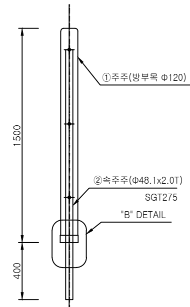
로프형 목재휨스 1500 KD-LOB-W1500 (H1.5xW1.5)
