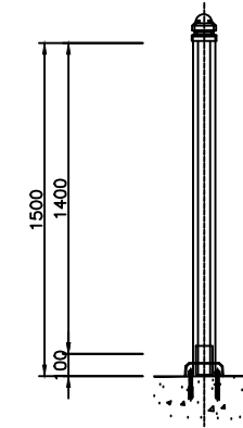
SIDE VIEW SCALE: NONE
