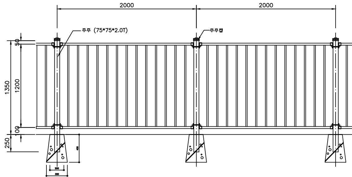
ELEVATION SCALE:NONE
