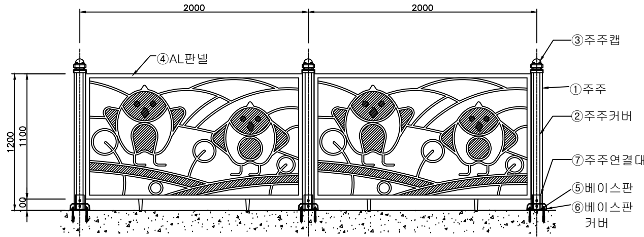
ELEVATION SCALE:NONE
