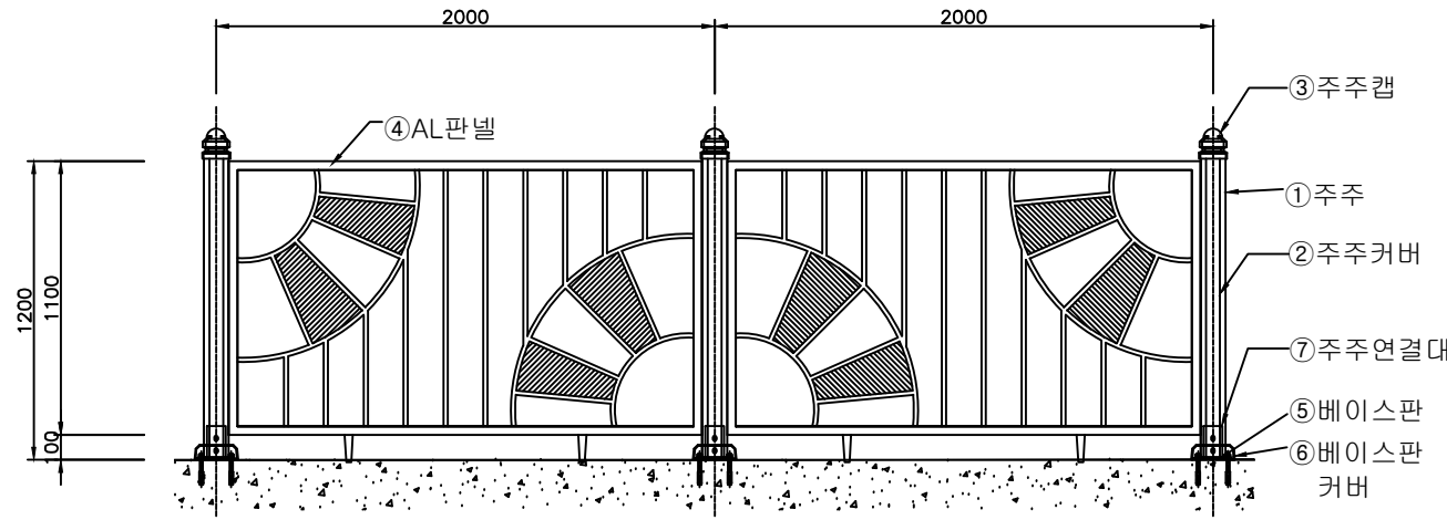
ELEVATION SCALE:NONE
