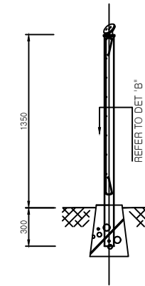
SIDE VIEW SCALE: NONE
