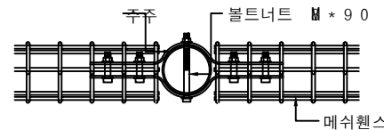
"B" DETAIL SCALE: NONE
