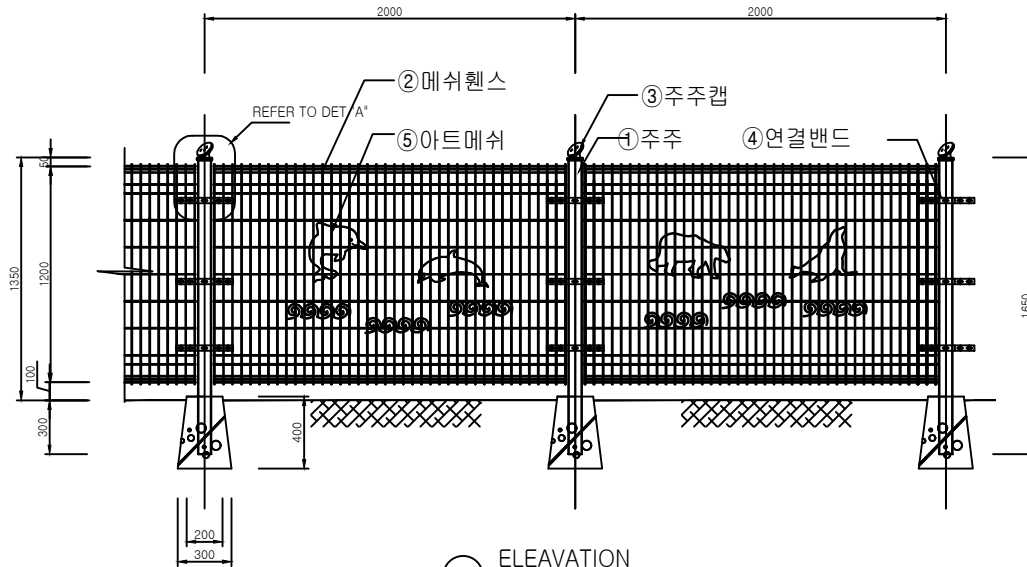
ELEVATION SCALE: NONE
