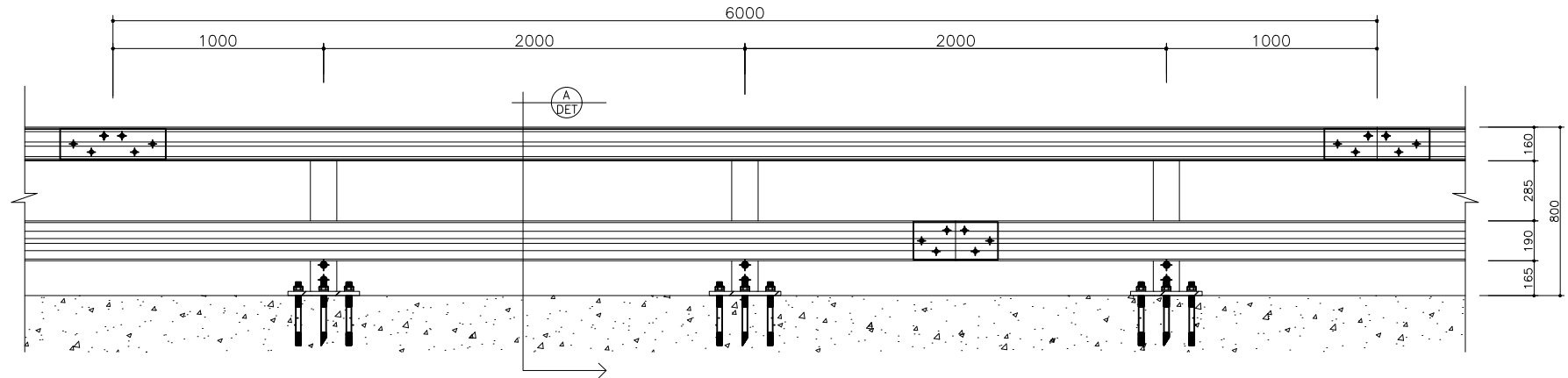
ELEVATION
