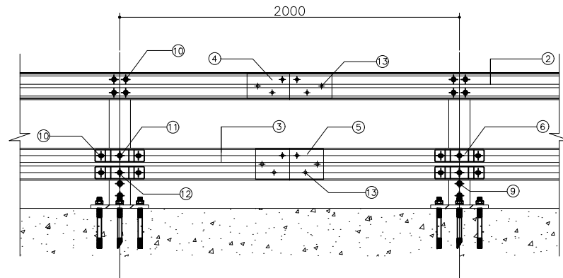
ELE "V" DETAIL
