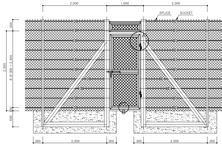
입면도
