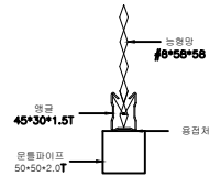
B 상세도
