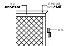
A 상세도
