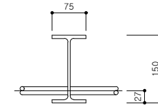
H-BEAM 상세
