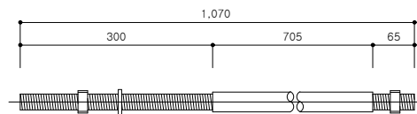
SPLICE 상세
