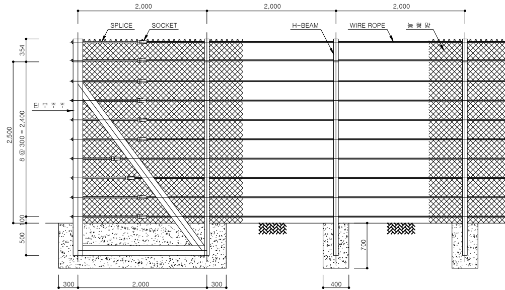
입면도
