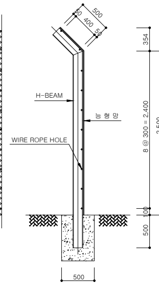
단면도
