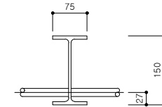
H-BEAM 상세
