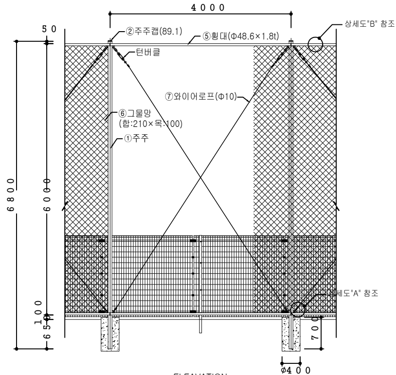
ELEVATION SCALE: NONE
