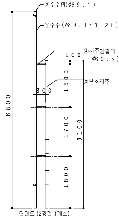
단면도 (2경간 1개소)
