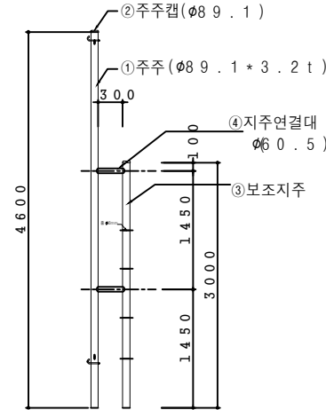
단면도 (2경간1개소)
