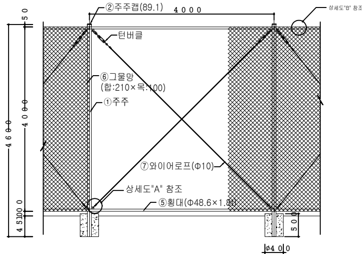
ELEVATION SCALE: NONE
