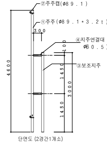
SIDE VIEW SCALE: NONE
