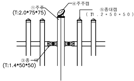
"A" DETAIL SCALE: NONE
