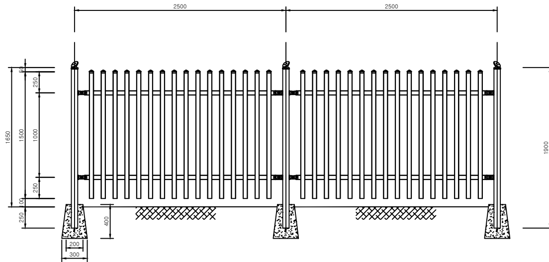
ELEVATION SCALE: NONE
