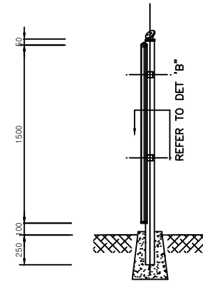
SIDE VIEW SCALE: NONE
