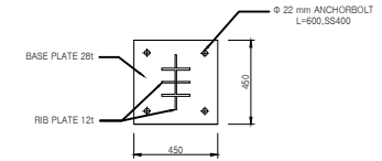
SET양카용 베이스 플레이트 상세도
