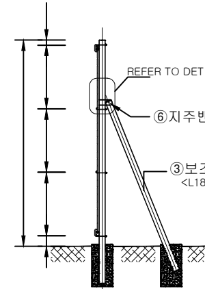
SIDE VIEW SCALE: NONE
