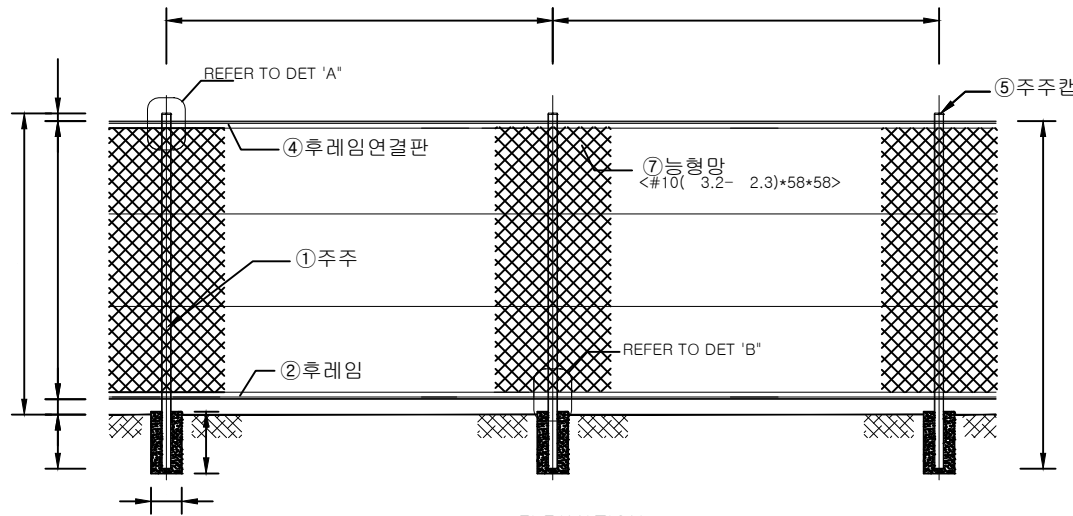
ELEVATION SCALE: NONE
