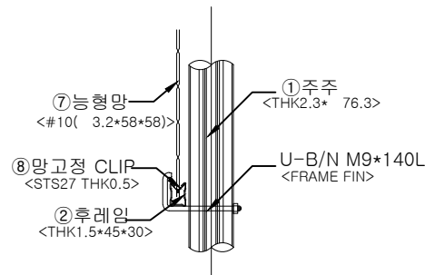
"B" DETAIL SCALE: NONE
